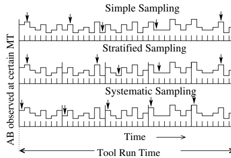
Fig. 2. Sampling Strategies
