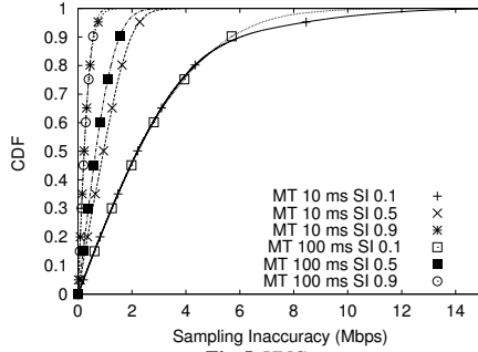
Fig. 5. UNC
