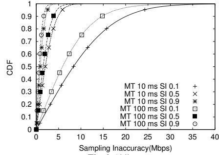
Fig. 6. Abilene
